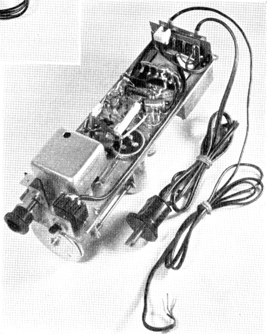
9. FM-tillsats enligt schemat i fig. 8 med avtagen kåpa, sedd ovanifrån.
