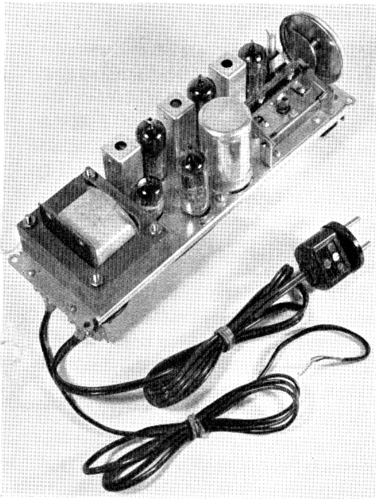
9. FM-tillsats enligt schemat i fig. 8 med avtagen kåpa, sedd ovanifrån.
