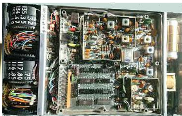
Ovanifrån öppnad
