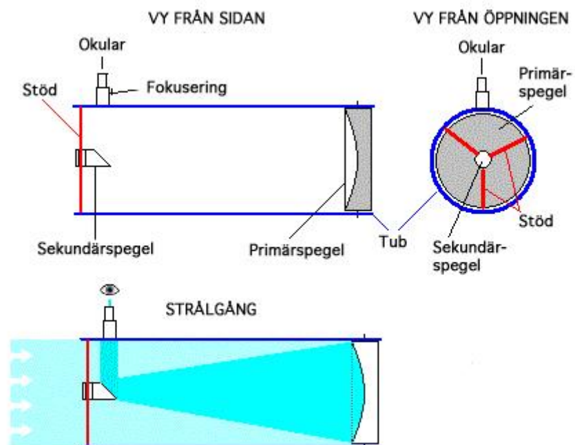
Bild över hur ett Newtonteleskop fungerar (Wikipedia).
