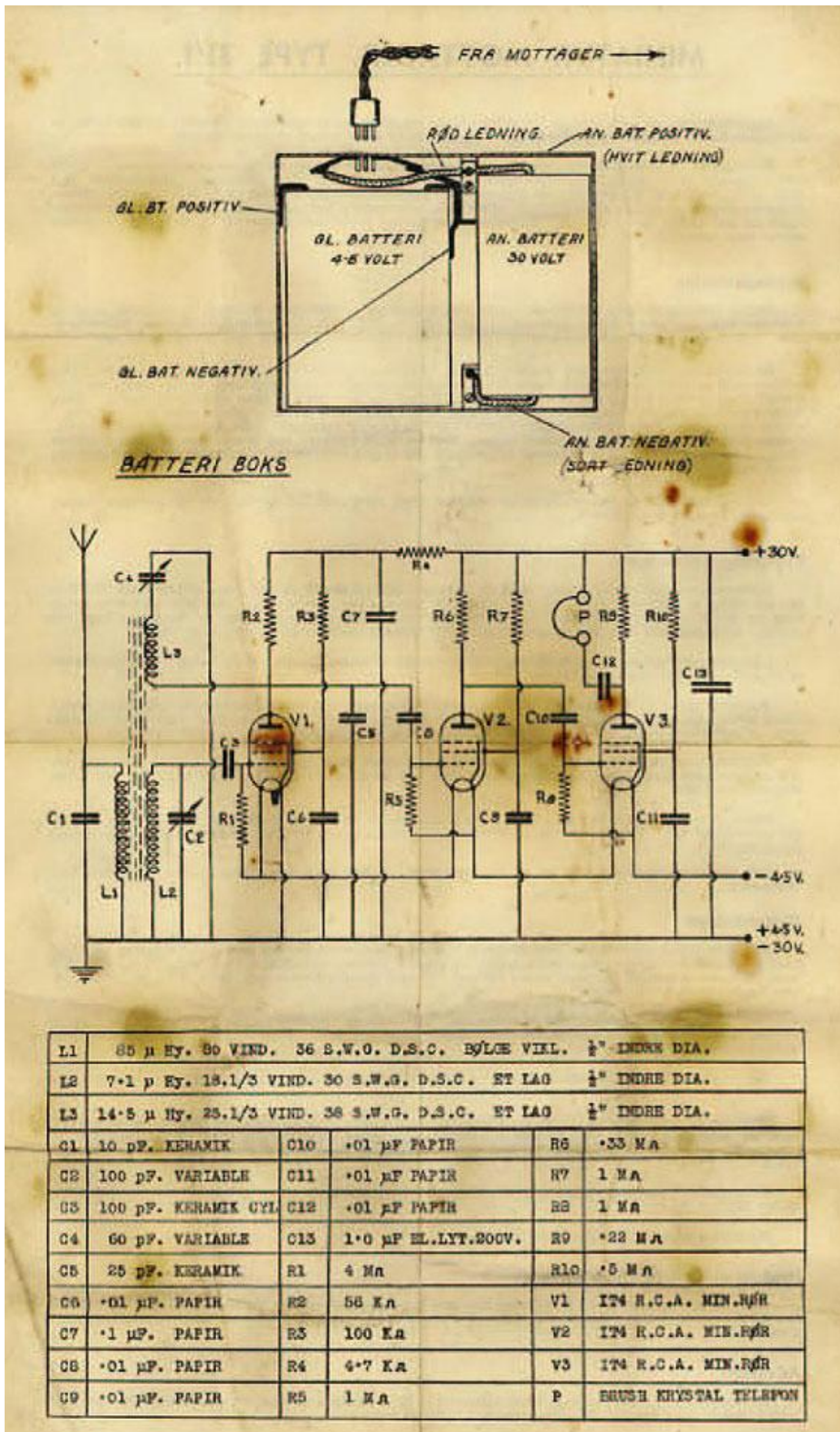
Kopplingschema och komponenter till Sweetheart.
